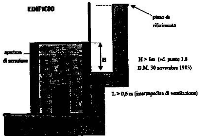
tavola 2 a - locale interrato
