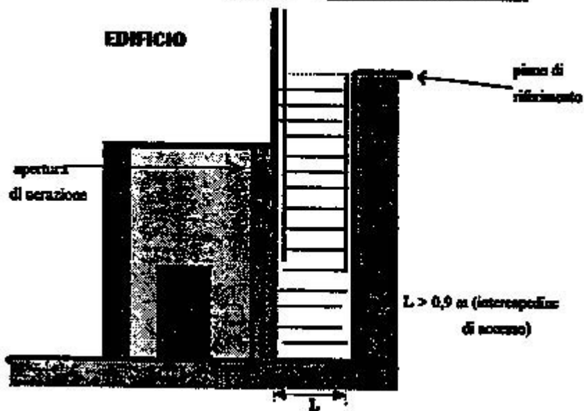
tavola 2 b - locale interrato
