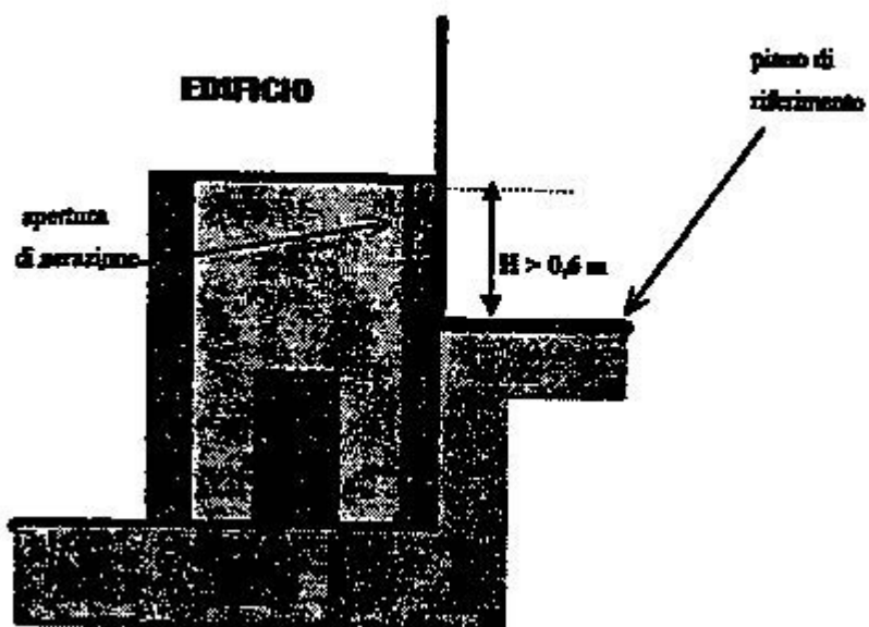
Tavola 4 - installazione all'aperto in adiacenza a parete
